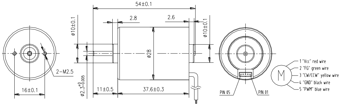
※ 电机主要技术参数 Motor Technical Data
