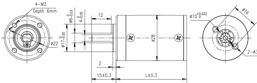
※ 配置电机的完整型号:FBL-2838HRX□( □内填写减速比)
