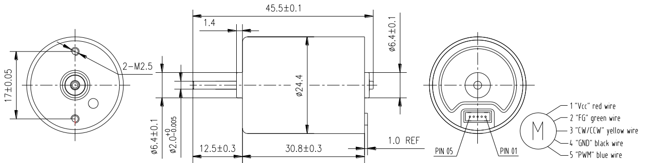
※ 电机外形尺寸 Motor Overall Dimension
