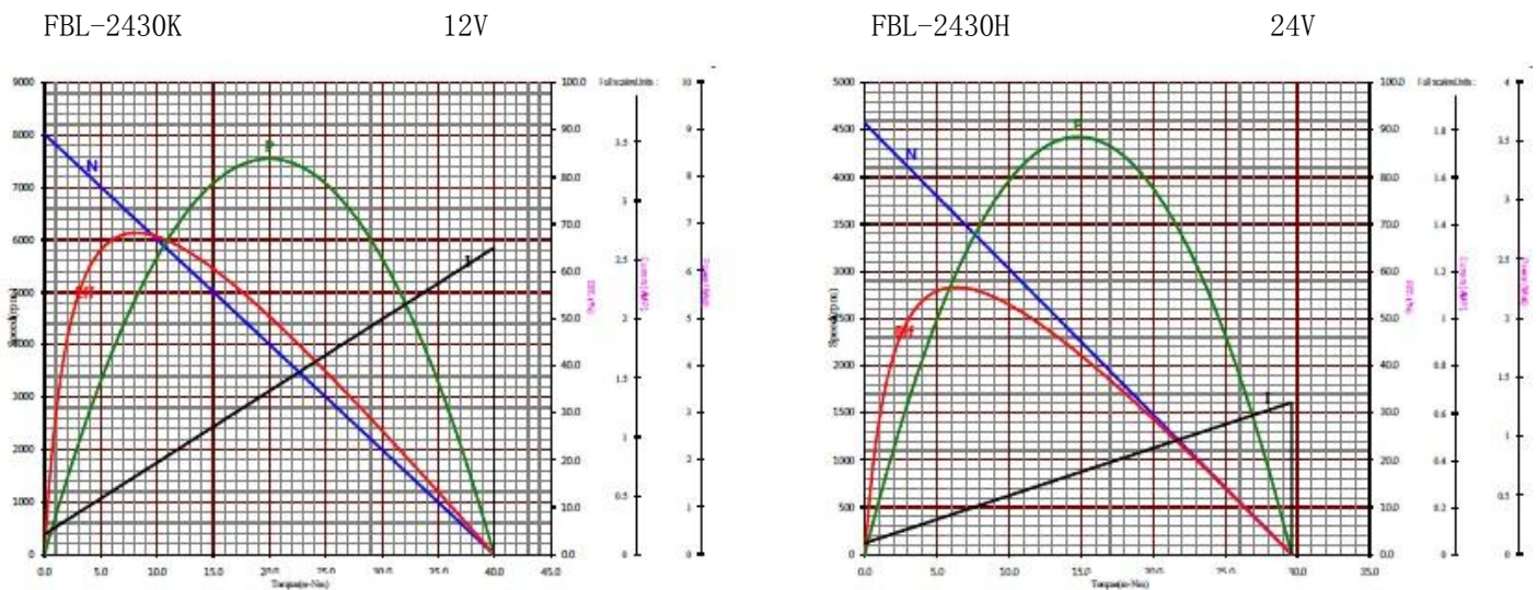
※ 性能曲线 Performance Curve
