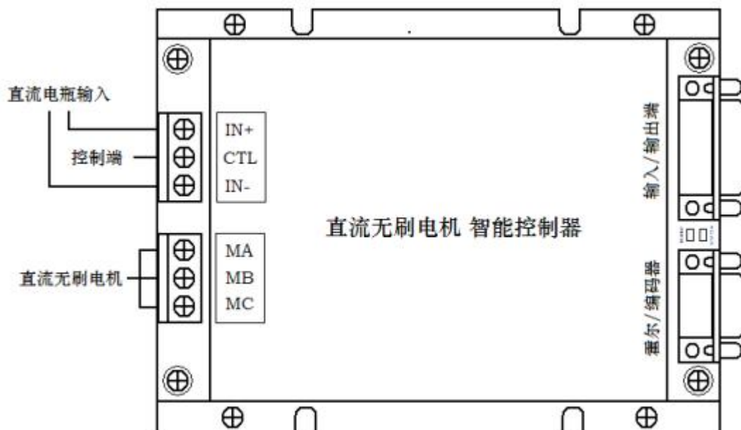
接线端子说明
