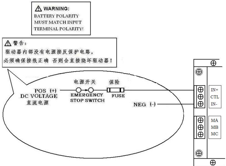
保险、电源开关的连接图
