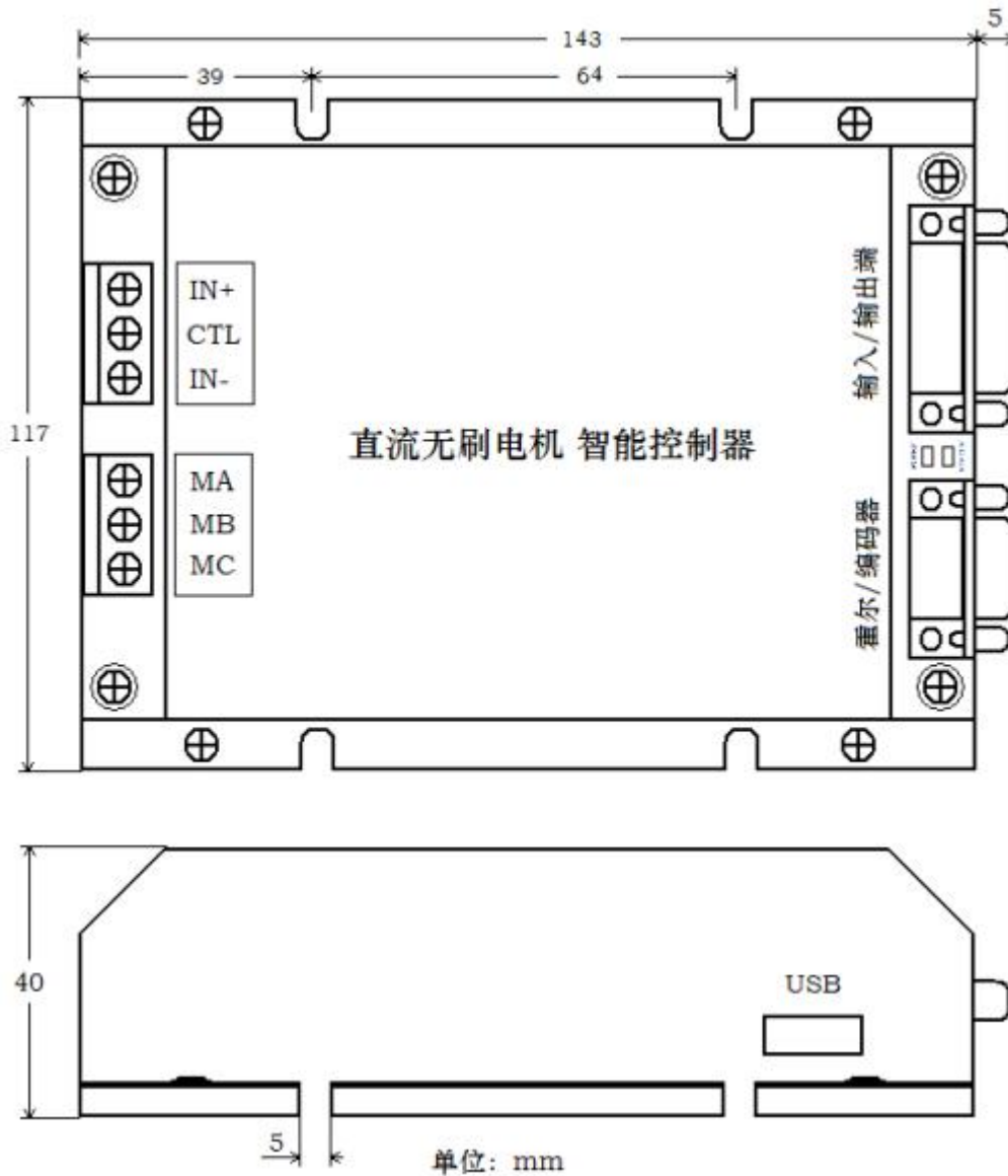
外形尺寸图
